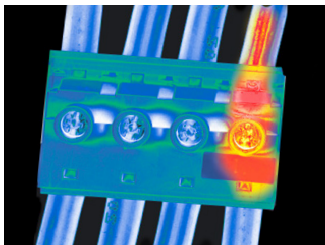
Überlastung des Neutralleiters
