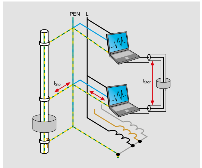
EMV- ungünstiges TN-C System (4 Leiter)
